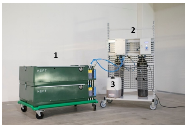
Figuur 2.10: Het materiaal bestaat uit een of meerdere boxen (1) met schuimgeneratoren, een stikstofunit (2) en schuimoplossing (3). Bron foto: RASA
