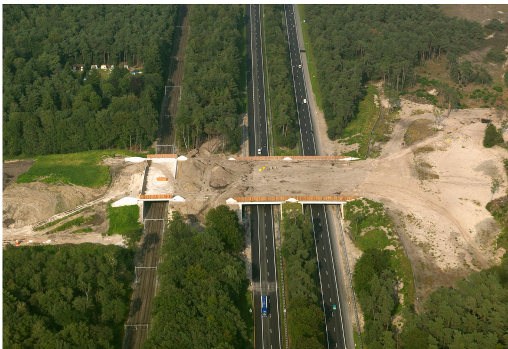
Figuur 3.1 Aanleg ecoduct Hulshorst over bestaande weg en spoorweg (foto: Combinatie H 2 Eco).
