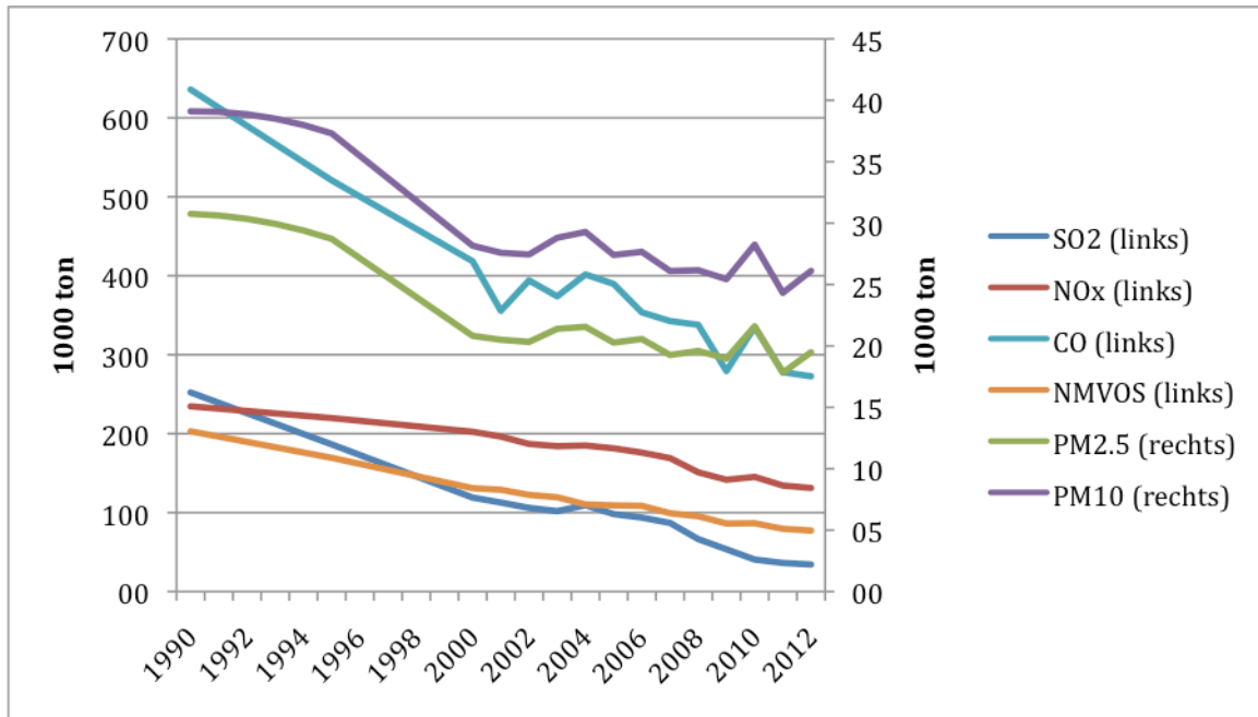
Figuur 14: Emissies naar de lucht in Vlaanderen (luchtverontreiniging)
