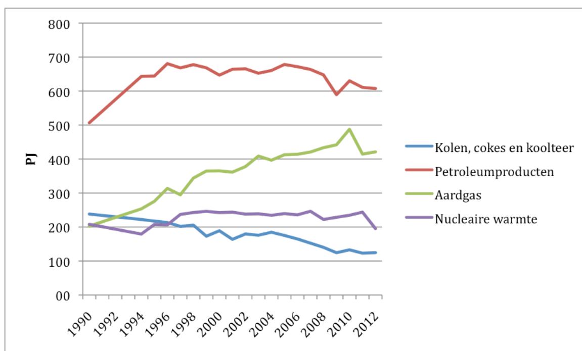
Figuur 18: Energieconsumptie in Vlaanderen
